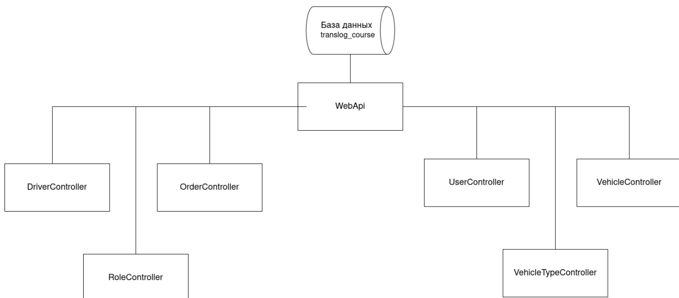
Рисунок 2.1.2 – Модульная схема WebApi
